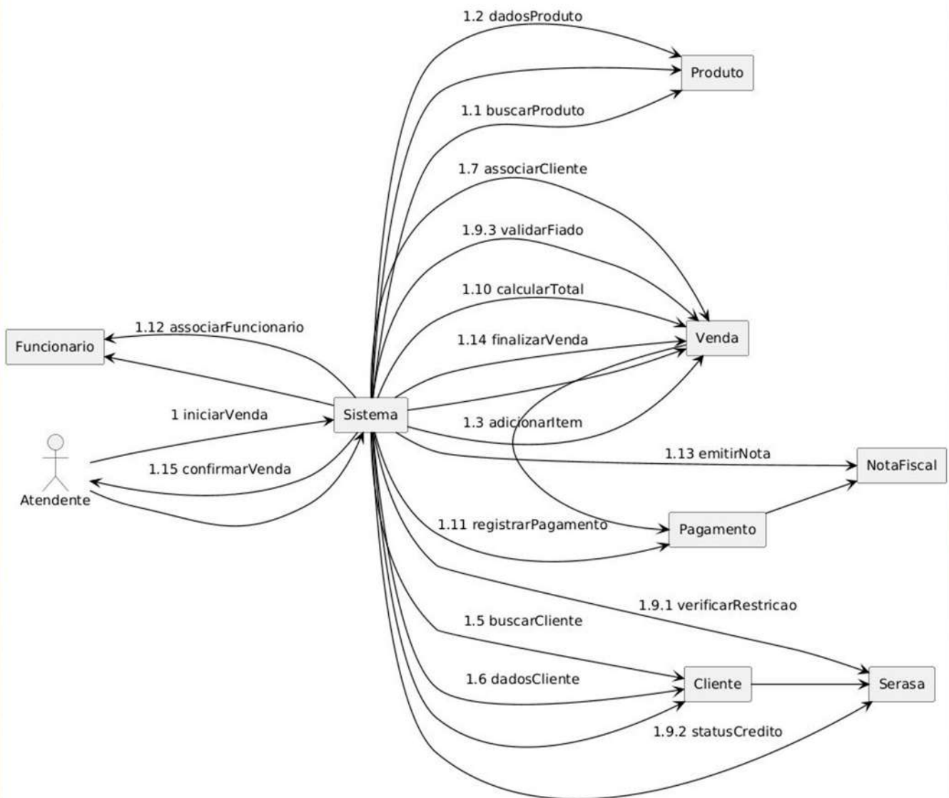
Diagrama de Comunicação / Colaboração Cenário: Realizar Venda (Fluxo Principal)
